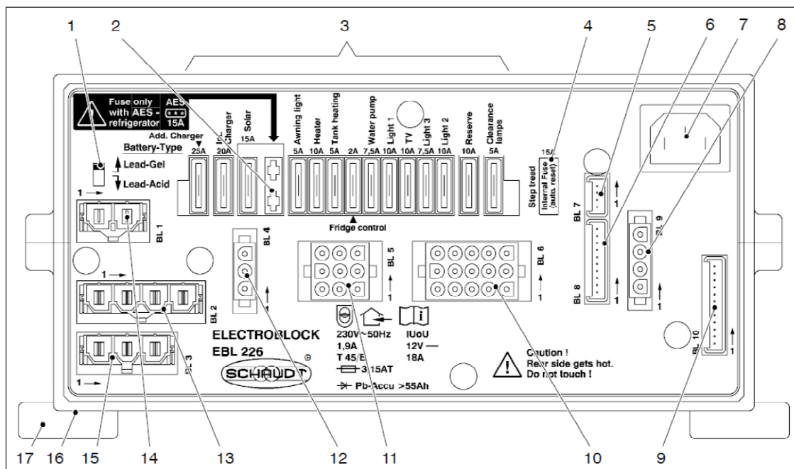
Bild 4 Aufbau Elektroblock EBL 267 a (Front)
