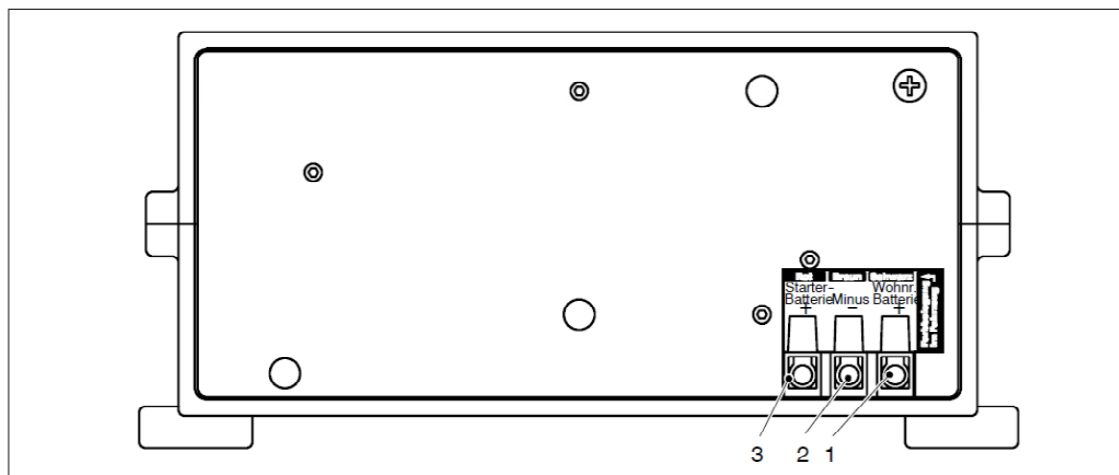
Bild 5 Aufbau Elektroblock EBL 267 a (Rückseite)
